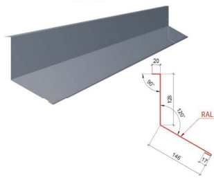
Планка примикання ТИП 1
