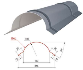
Планка конька напівкругла
