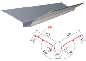
Планка примикання ТИП 1
