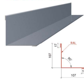
Планка кутова внутрішня ТИП 1
