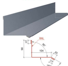
Планка примикання ТИП 2
