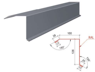
Планка розжолобка нижня ТИП 2
