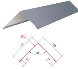
Планка вітрова ТИП 1
