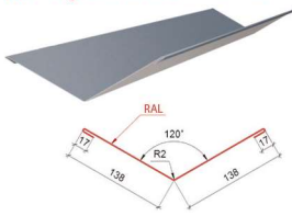
Планка примикання ТИП 2
