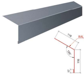
Планка розжолобка декоративна ТИП 2
