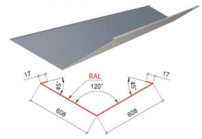
Планка кутова зовнішня ТИП 1
