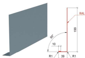
Планка лобова ТИП 1
