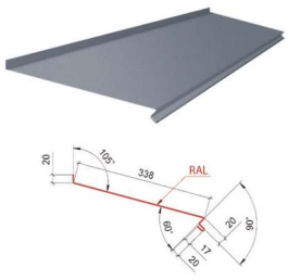
Планка лобова ТИП 1
