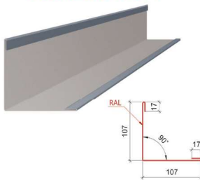
Планка кутова зовнішня ТИП 1
