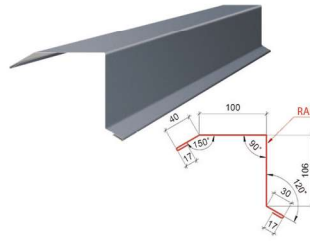
Планка розжолобка нижня ТИП 1
