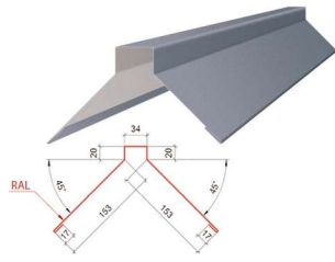
Планка карнизна ТИП 2
