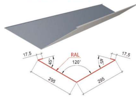
Планка кутова внутрішня ТИП 1
