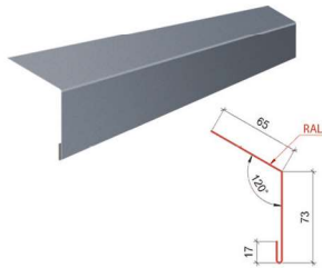
Планка розжолобка декоративна ТИП 1
