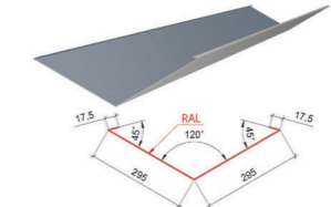
Планка кутова внутрішня ТИП 1
