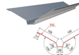
Планка примикання ТИП 1
