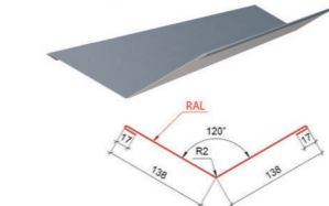
Планка примикання ТИП 2
