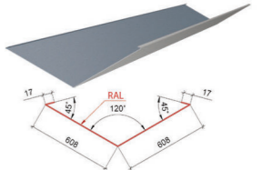
Планка кутова зовнішня ТИП 1
