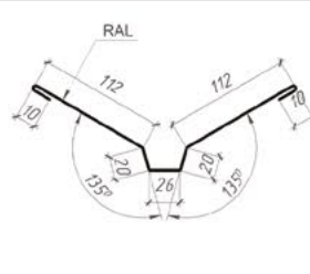
Планка розжолобка нижня Тип 1 Ширина штрипса 625 мм
