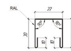
Планка П-подібна С-18, С-20 Ширина штрипса 102 мм
