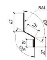
Планка вирівнююча Тип 1
