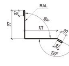
Планка кутова зовнішня Тип 2 Ширина штрипса 250 мм
