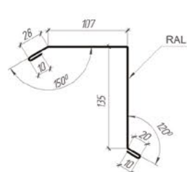
Планка розжолобка декоративна Тип 1 ШІРИНА ШТРИПСА 312 мм
