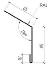
Планка вітрова Тип 2 ШИРИНА ШТРИПСА 312 мм
