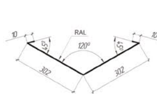
Планка розжолобка нижня Тип 4 Ширина штрипса 416 мм
