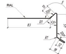
Планка під бітум Ширина штрипса 178 мм
