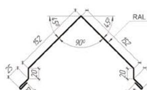
Планка карнизна Тип 2
