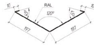
Планка розжолобка нижня Тип 4 Ширина штрипса 416 мм
